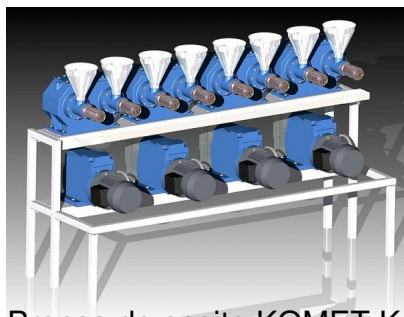
Prensa de aceite KOMET K 120 I
